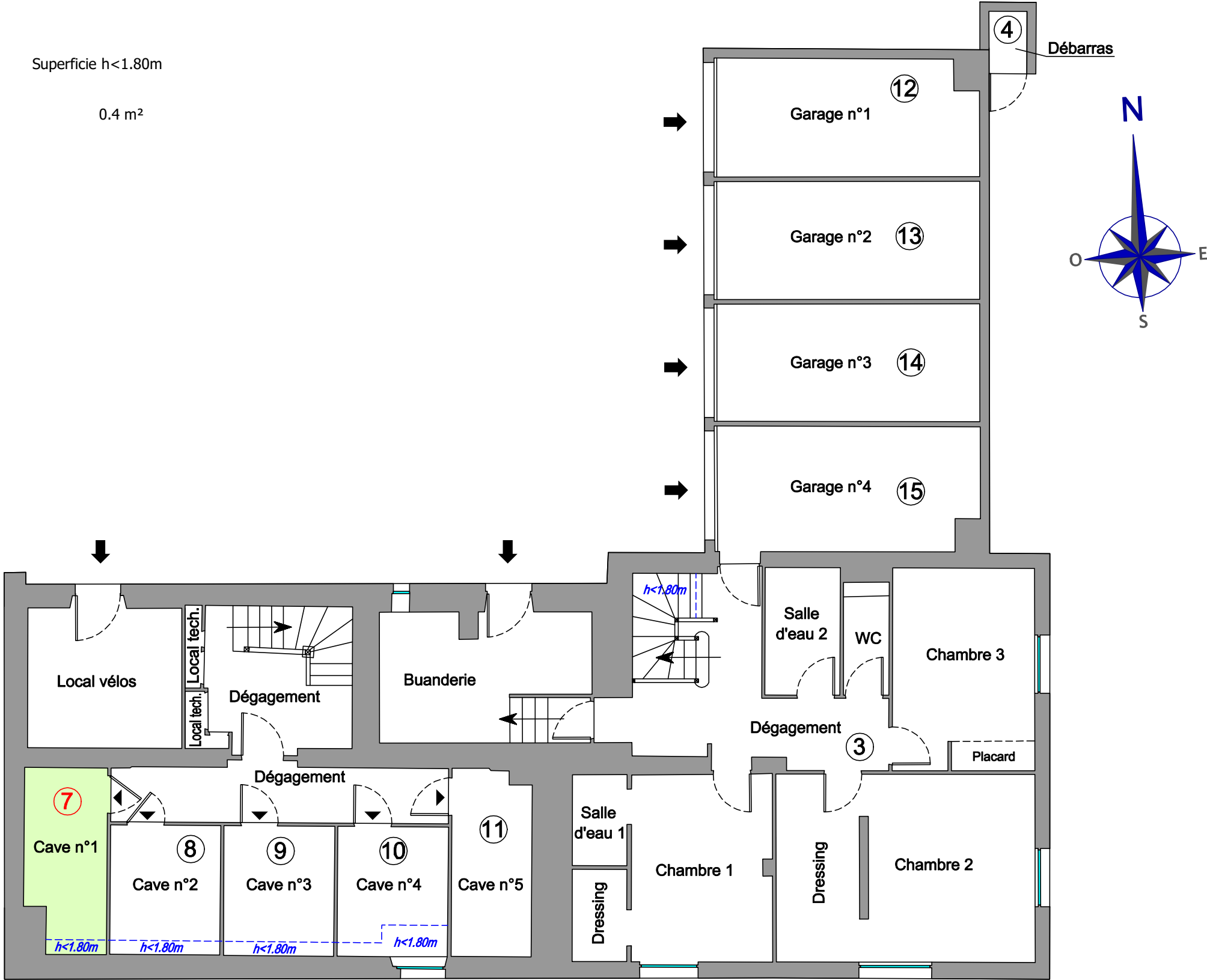
Rez-de-jardin
